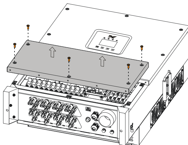
Rysunek 3-20 Zdemontować pokrywę.
