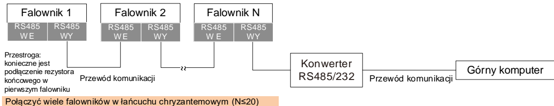
Rysunek 3-27 System komunikacji wielu falowników
