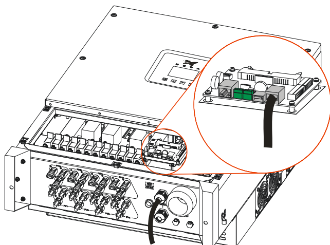
Rysunek 3-29 Złącze komunikacji DRM
